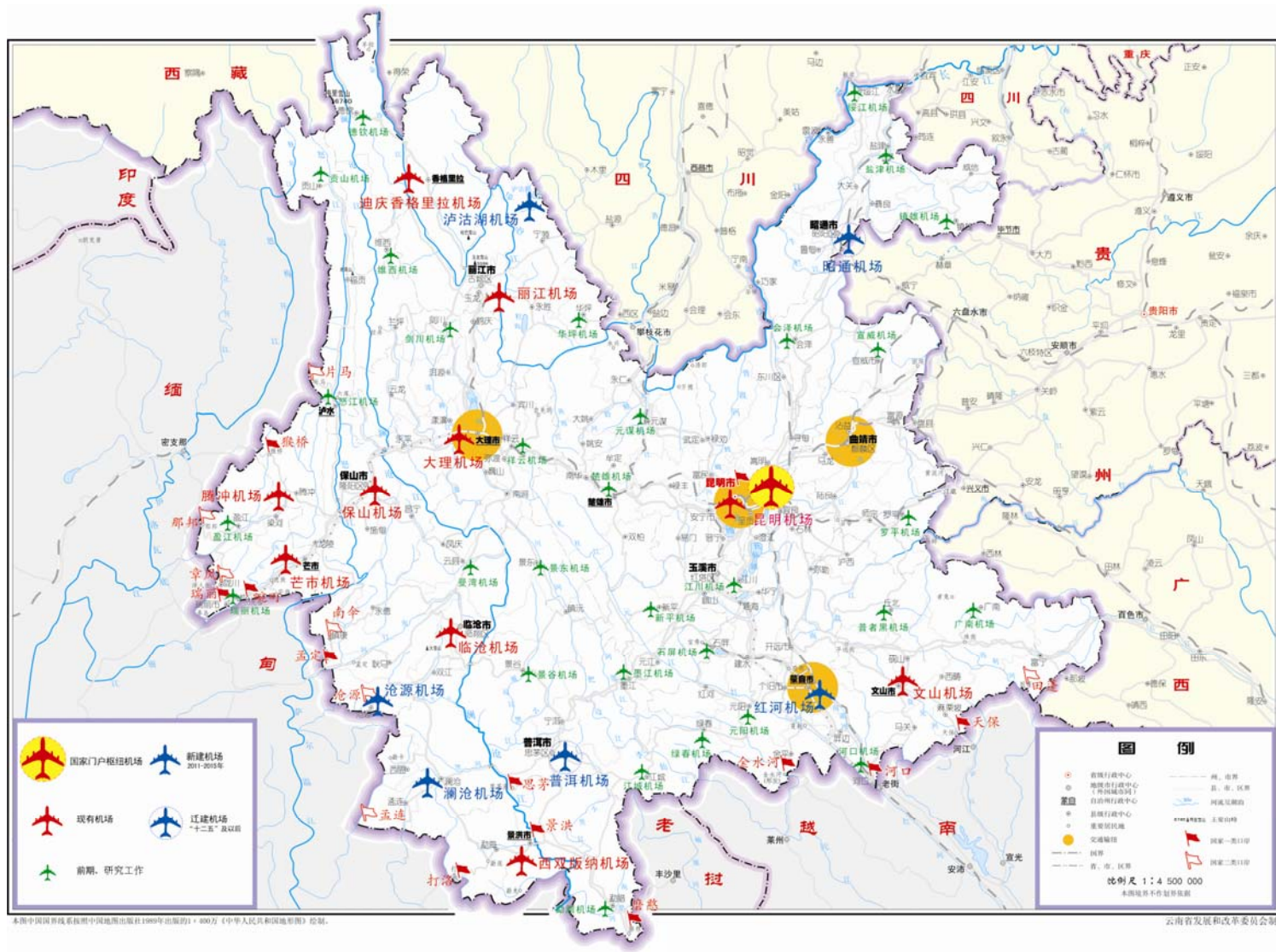
附图 6 云南省“十二五”及中长期机场布局规划图
